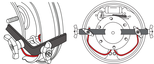
2007 SILVERADO HUB
