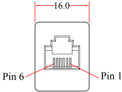
RJ12 Jack1
