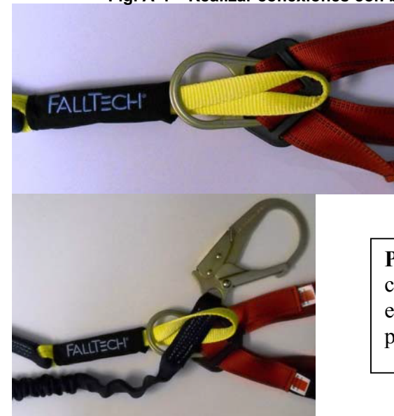
Fig. A-4 – Realizar conexiones con bucle de fijación
