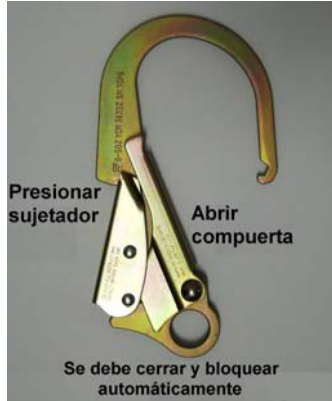
Fig. A-2 – Gancho de refuerzo
