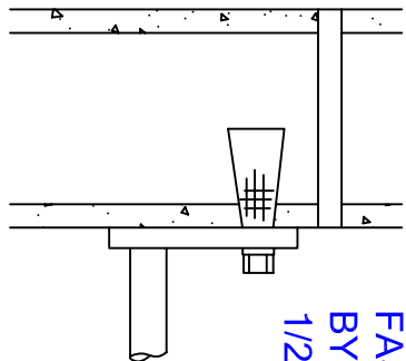
DETAIL A-A
