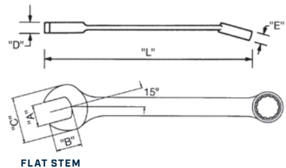
FLAT STEM
