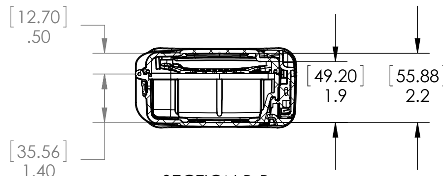
SECTION B-B SCALE 1 : 3
