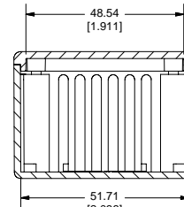
SECTION D-D
