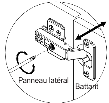
AJUSTEMENT - AJOUR
