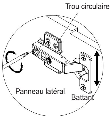
AJUSTEMENT - HAUTEUR
