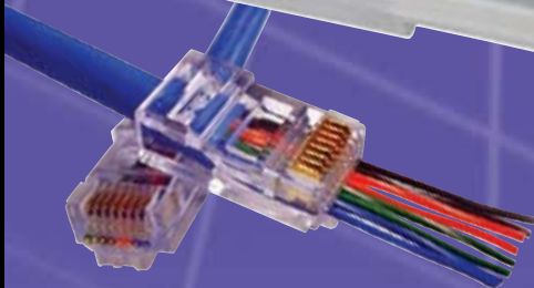
EZ-RJ45 Cat5e connector P/N 105003
