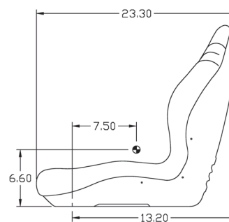
SIDE VIEW PN: 6831
